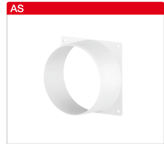
■ Anschluss-Stutzen AS Mit quadratischer Flanschplatte (102 x 102 mm) und rundem Stutzen (50 mm lang), aus Kunststoff. Zum Aufsetzen von Rohren (ND 100) auf plane Flächen.
