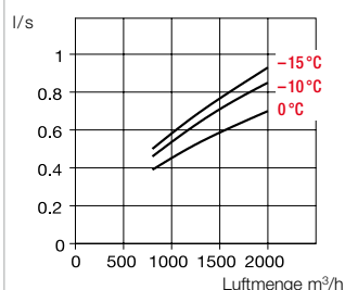
④ Wasserdurchfluss bei 70/50 °C 1)
