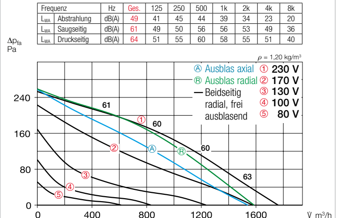
Ⓐ Ausblas axial Ⓑ Ausblas radial — Beidseitig radial, frei ausblasend
