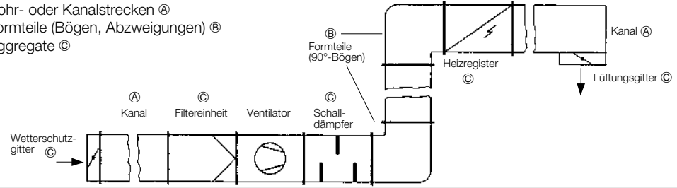
Bild 9 Druckverluste in einer Lüftungsanlage
