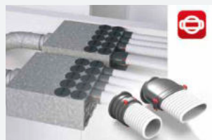
Die Verteilerkästen können mit runden und ovalen Einzelstutzen sowie mit einer Mischbelegung bestückt werden.
