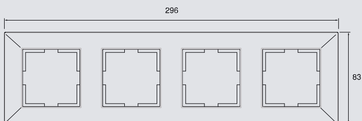
4-fach Rahmen
