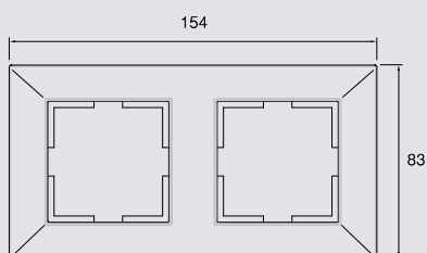
2-fach Rahmen
