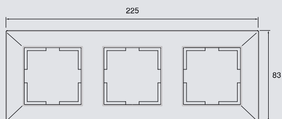
3-fach Rahmen
