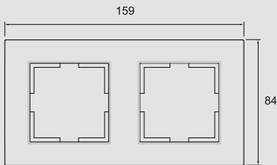
2-fach Rahmen
