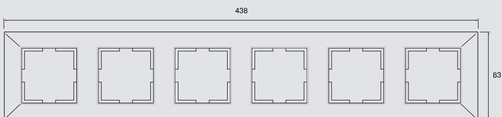
6-fach Rahmen
