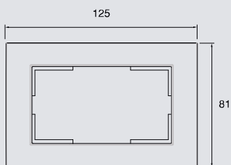
Rahmen Doppelsteckdose
