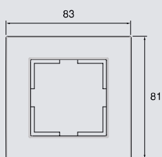
1-fach Rahmen
