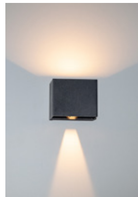
Abstrahlwinkel oben: 120° Abstrahlwinkel unten: 30°
