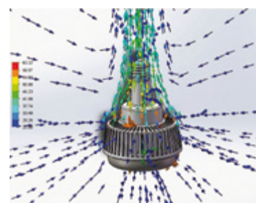
Innovativer COOLFIN Kühler mit Kamin-effekt in Leichtbauweise
