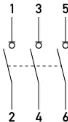
Anschlussschema
