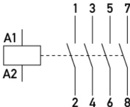
Anschlussschema
