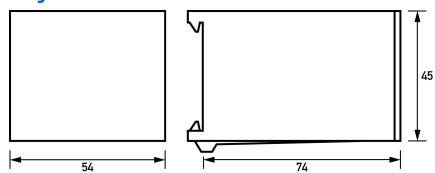
Maßzeichnung Gruppenansicht
