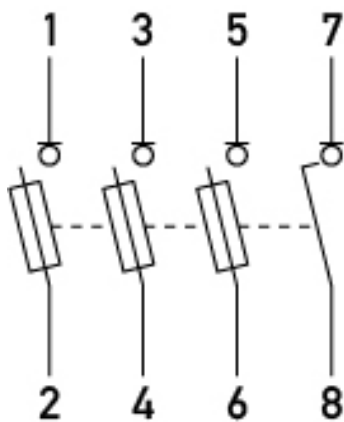
Anschlussschema
