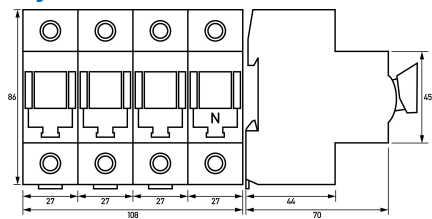
Maßzeichnung Gruppenansicht
