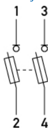
Anschlussschema
