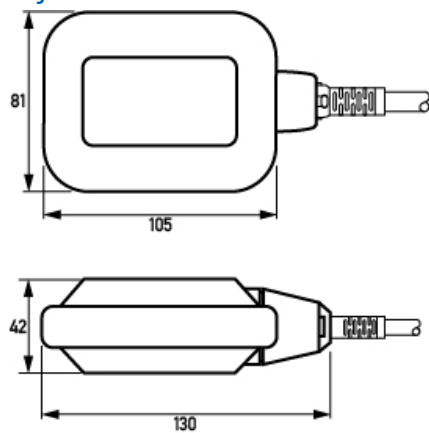
Maßzeichnung Gruppenansicht
