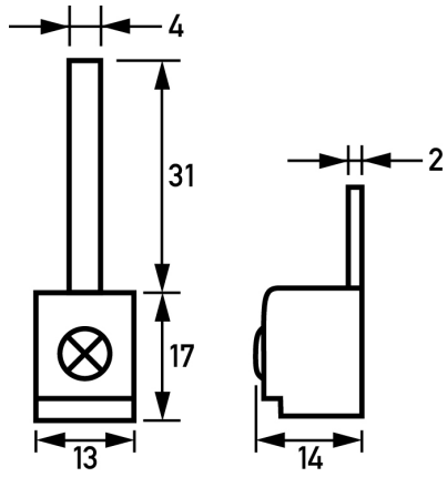
Maßzeichnung Gruppenansicht
