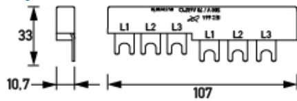
Maßzeichnung Gruppenansicht
