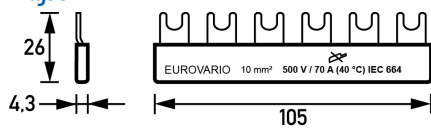
Maßzeichnung Gruppenansicht
