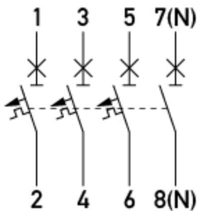
Anschlusschema
