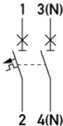
Anschlusschema
