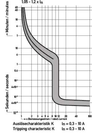
Kennlinie Char. K
