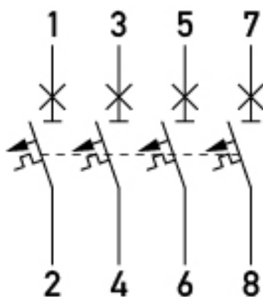
Anschlussschema
