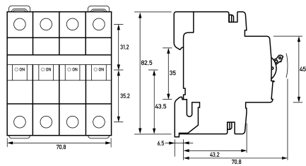
Maßzeichnung Gruppenansicht
