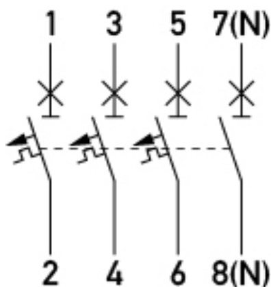
Anschlusschema
