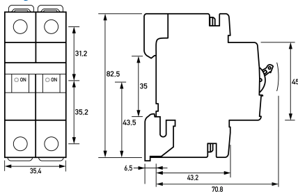
Maßzeichnung Gruppenansicht
