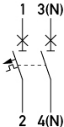
Anschlussschema
