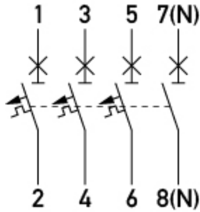
Anschlusschema
