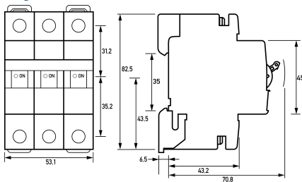
Maßzeichnung Gruppenansicht
