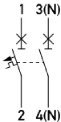
Anschlussschema
