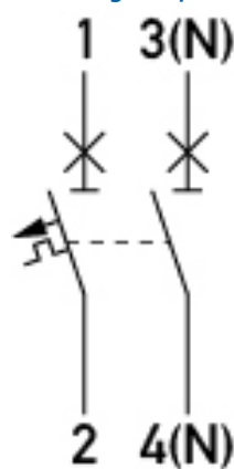
Anschlusschema
