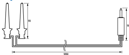
Maßzeichnung Gruppenansicht
