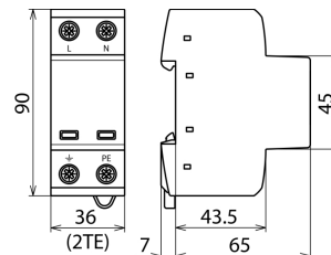
Maßbild DSH TT 2P 255
