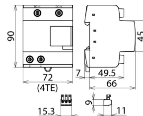
Maßbild DCB YPV SCI 600 FM
