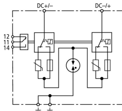
Prinzipialschaltbild DCB YPV SCI 600 FM
