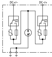
Principalschaltbild DCB YPV SCI 1500
