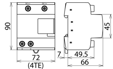
Maßbild DCB YPV SCI 1500
