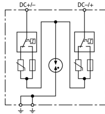
Prinzipialschaltbild DCB YPV SCI 600
