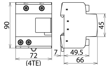
Maßbild DCB YPV SCI 600
