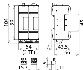
Maßbild DG SE PV SCI 1500 FM
