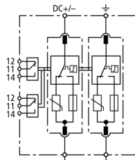
Prinzipschaltbild DG SE PV SCI 1500 FM
