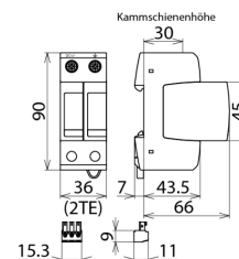
Maßbild DG S PV SCI 600 FM
