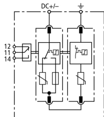
Prinzipialschaltbild DG S PV SCI 600 FM
