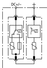
Prinzipialschaltbild DG S PV SCI 600
