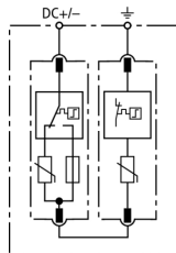
Prinzipialschaltbild DG S PV SCI 150
