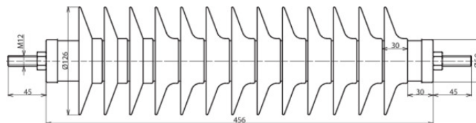
Maßbild DMI 51 10 1 H
