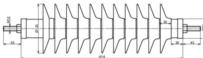
Maßbild DMI 45 10 1 H
