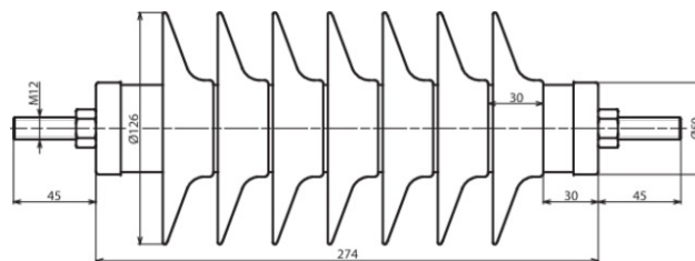
Maßbild DMI 33 10 1 H
