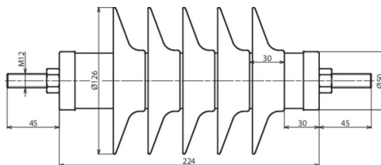
Maßbild DMI 24 10 1 H
