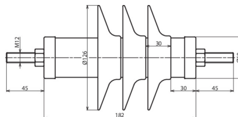
Maßbild DMI 18 10 1 H
