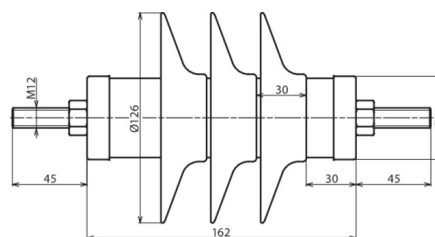
Maßbild DMI 15 10 1 H
