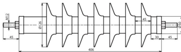
Maßbild DMI 42 10 1 N
