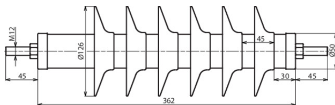
Maßbild DMI 36 10 1 N
