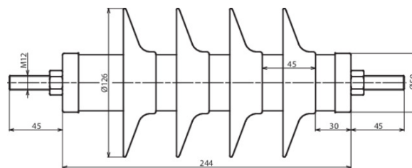
Maßbild DMI 27 10 1 N
