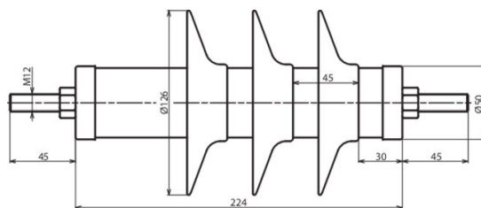
Maßbild DMI 24 10 1 N
