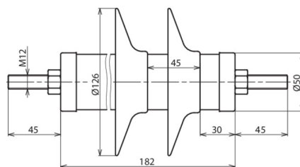
Maßbild DMI 18 10 1 N
