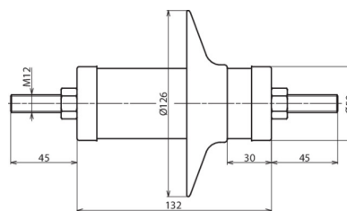
Maßbild DMI 9 10 1 N
