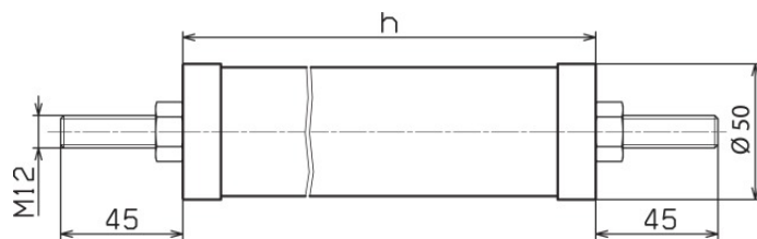
Maßbild DMI 39 10 1 L
