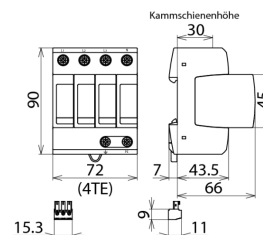
Maßbild DG M TT 150 FM
