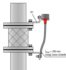
Einbauvariante EXFS L200
