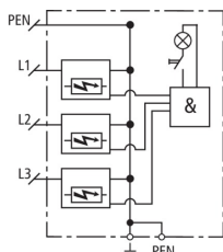
Prinzipialschaltbild DSH ZP TNC 255
