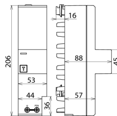
Maßbild DSH ZP TNC 255
