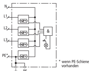
Prinzipialschaltbild DSH ZP B TT 255
