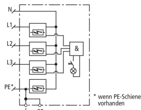
Prinzipschaltbild DSH ZP TT 255
