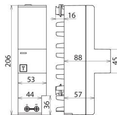
Maßbild DSH ZP TT 255
